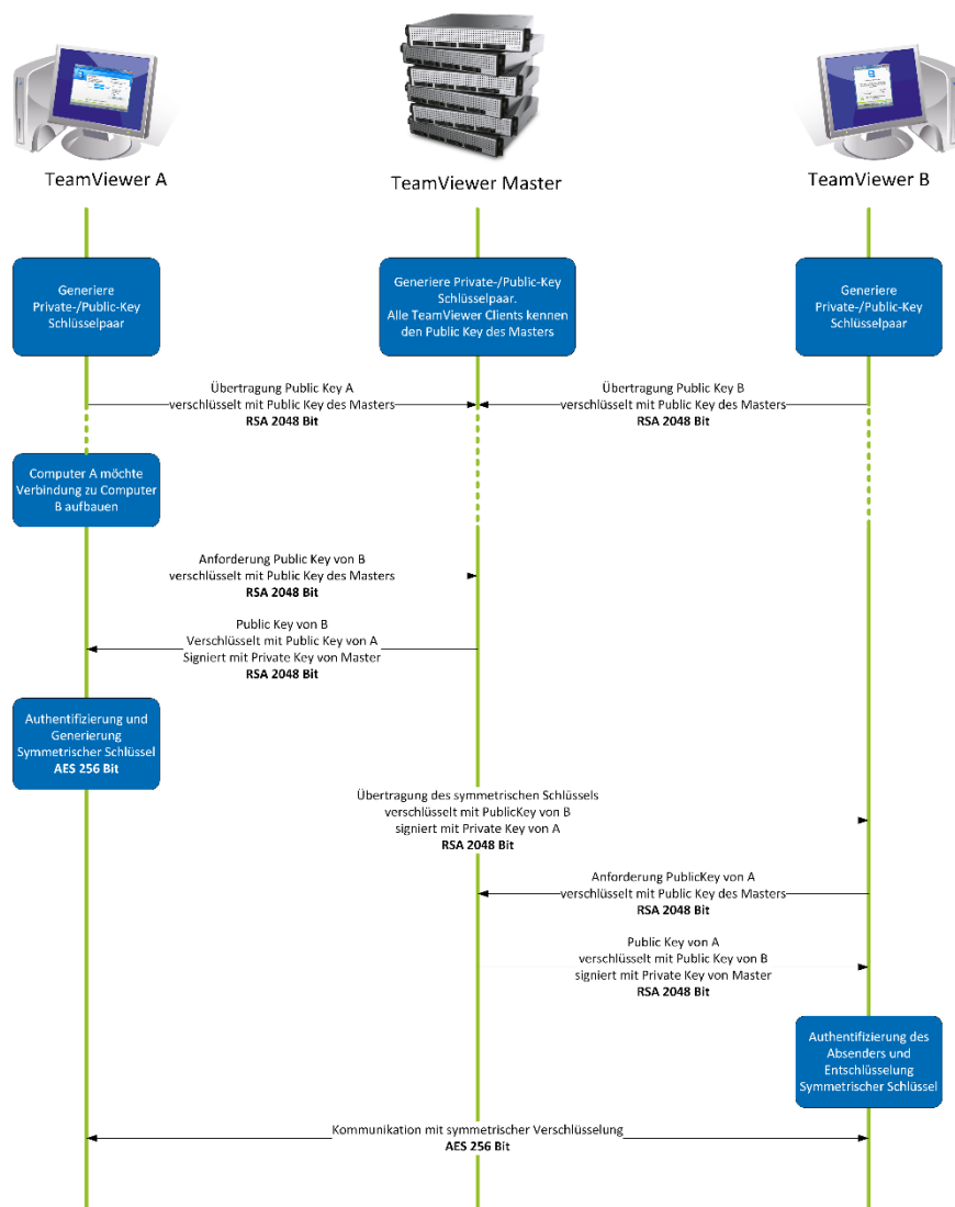
TeamViewer-Verschlüsselung und Authentifizierung
